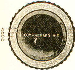
Den luftfyllda bollen. A. Luftbehållare. B. Hylsa till denna. C. Lager af öfvernystade trådar. D. Hård ytterhylsa.
