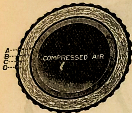
Den luftfyllda bollen. A. Luftbehållare. B. Hylsa till denna. C. Lager af öfvernystade trådar. D. Hård ytterhylsa.
